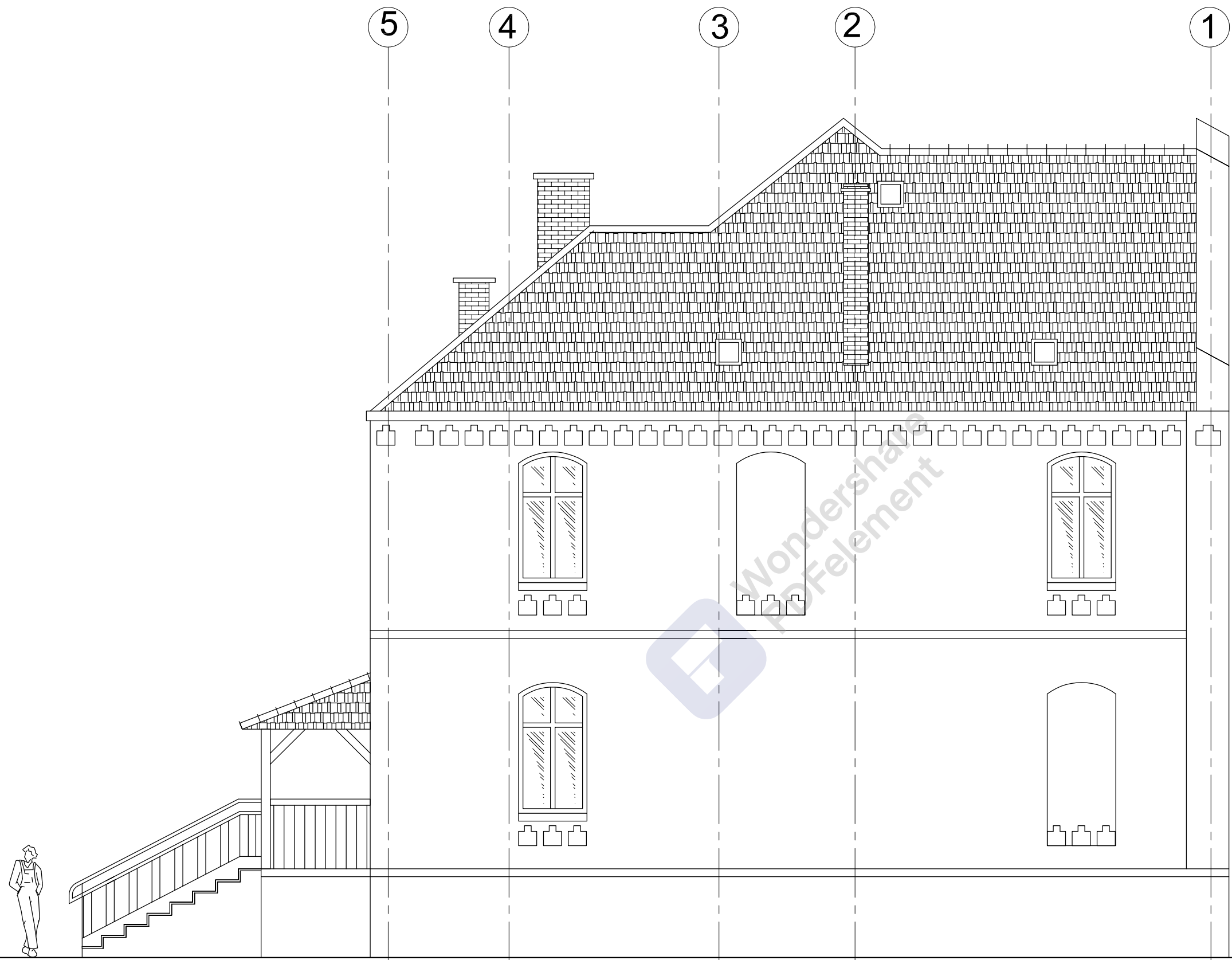
ELEWACJA ZACHODNIA skala 1:75
